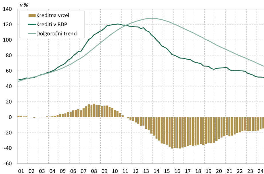
Slika 2: Kreditna vrzel
