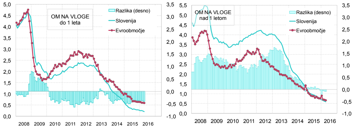
Slika 2: Primerjava slovenskih obrestnih mer z obrestnimi merami v evroobmočju za nove vloge gospodinjstev v odstotkih 1
